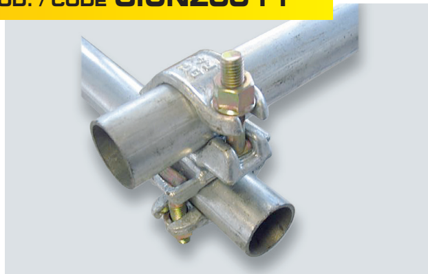
Giunto girevole tedesco a cerniera EN74
