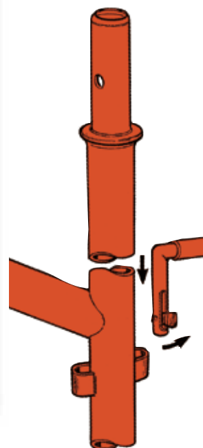
PARTICOLARE AGGANCI COUPLING PIN
